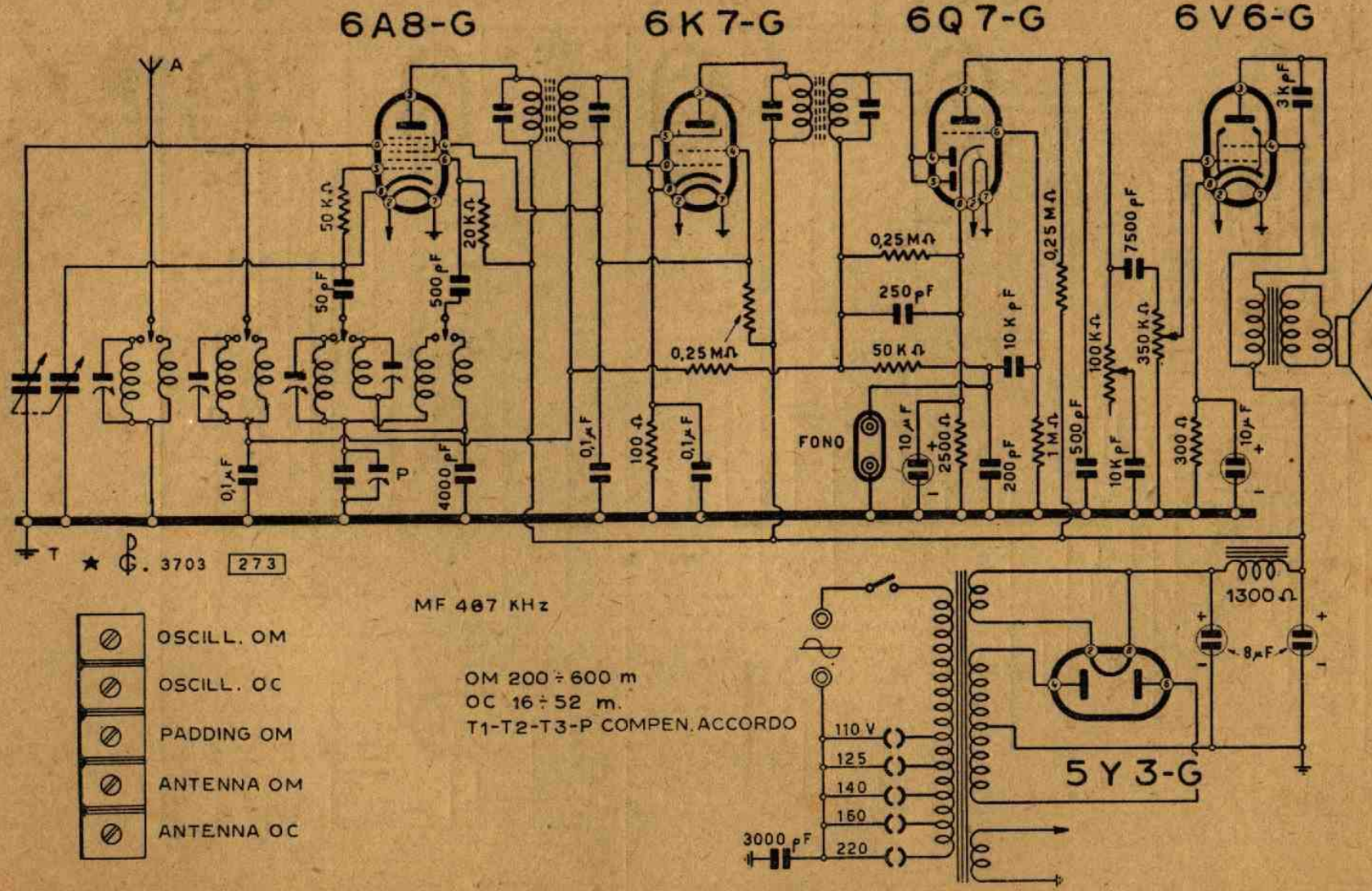
Lo schema elettrico del mod. 510 V. A. R. A.
